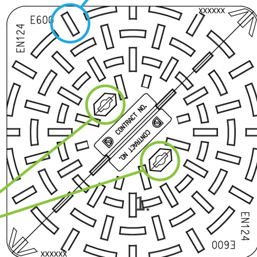
雨水渠渠蓋
