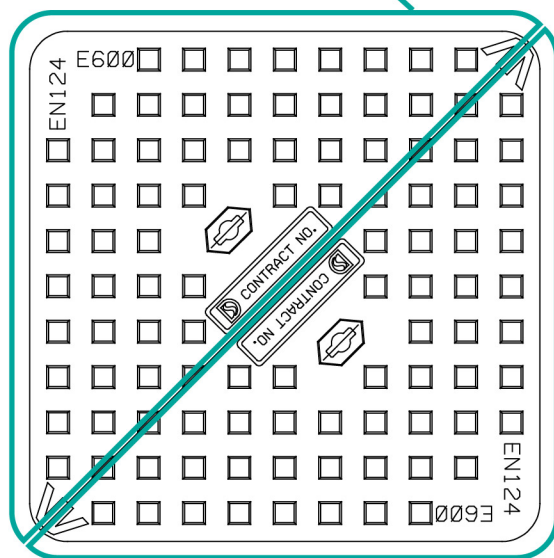
污水渠渠蓋
